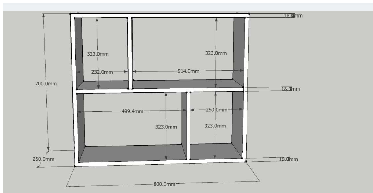
Скица 1: Зидна полица димензија 80x25x70 цм
