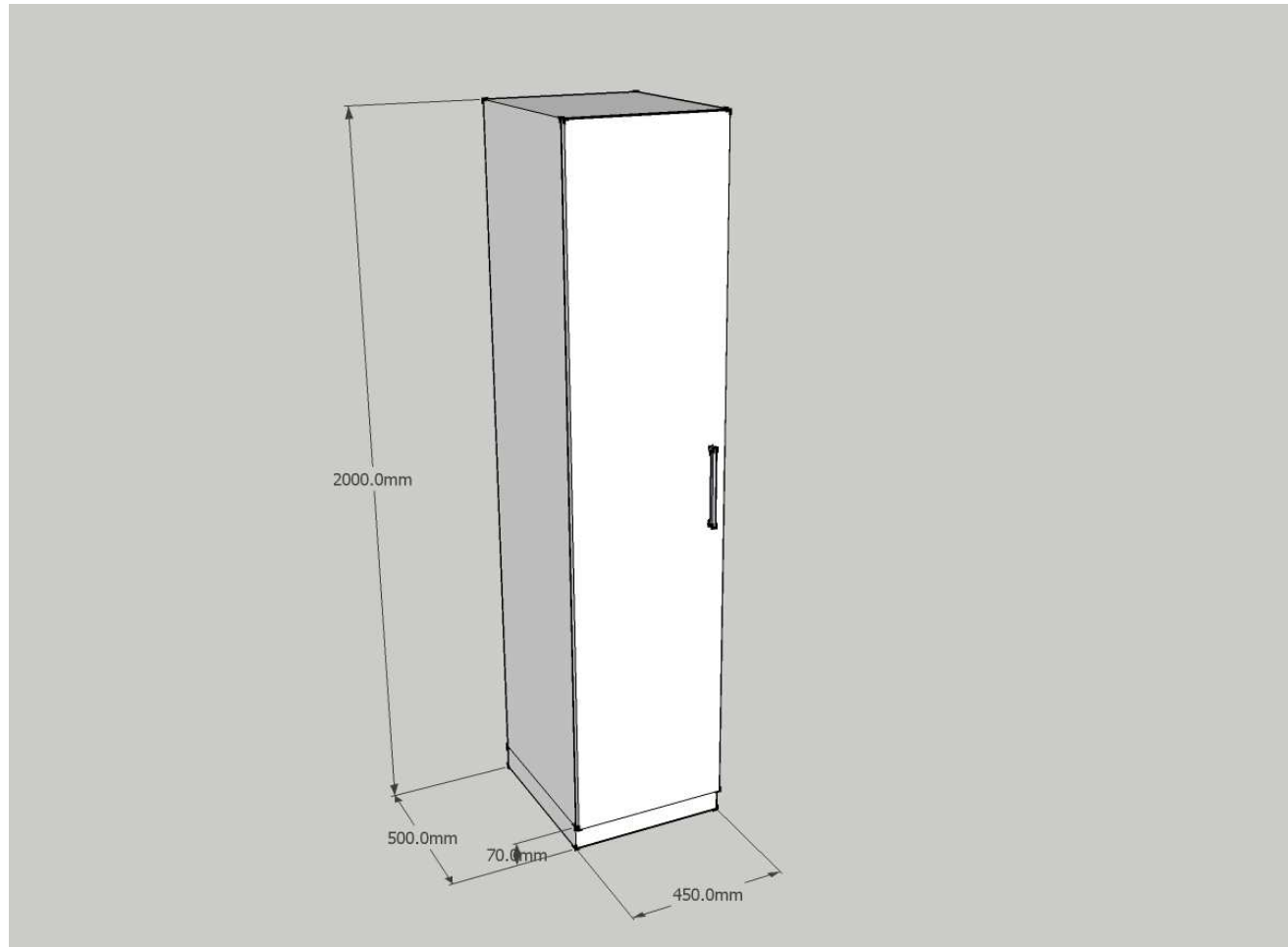
Скица 3: Ормар димензија 200x45x50 цм
