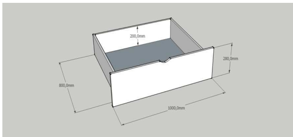
Скица 2: Фиока без ручица, димензија: 100x80x28 цм
